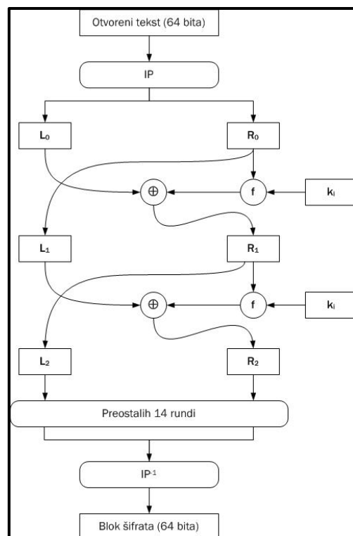
Slika 3. Feistelova mreža
